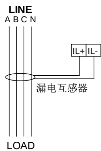
三相四线漏电互感器接线
