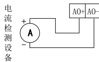
变送输出接线
