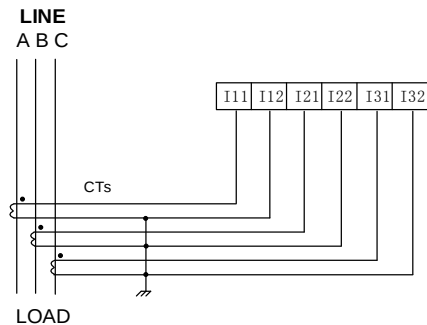
三相3CT
