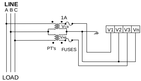
三相三线 2PT(V型,2LL)，高压
