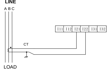
单相电流1CT
