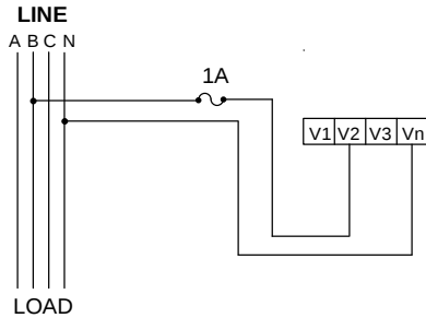
单相电压连接(3LN)
