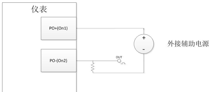
脉冲输出接线图（n 取 1-4）
