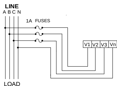
三相四线直接连接(3LN)，低压
