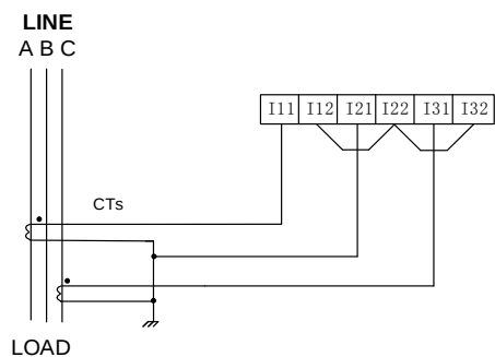
三相2CT (V型)
