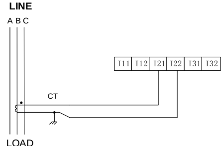
单相电流1CT
