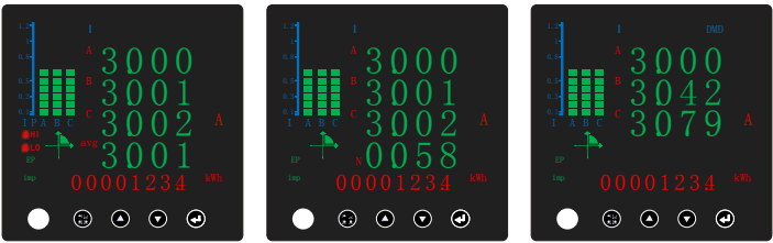
三相电流及均值 三相电流及中性线电流 三相电流需量
